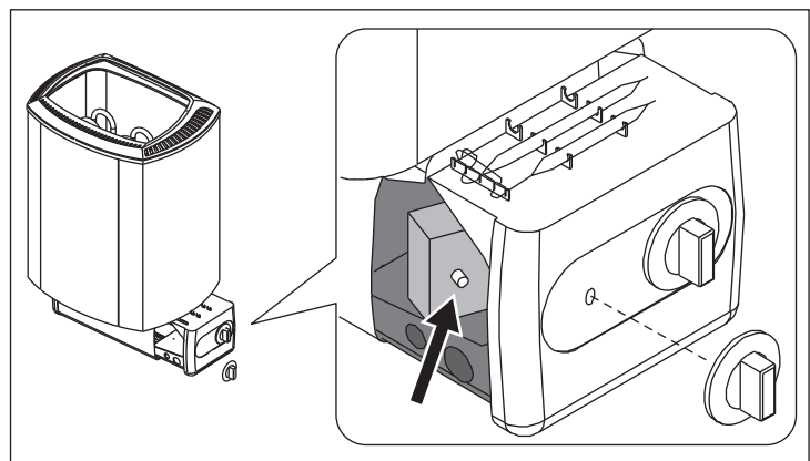
12. zīm. Pārkaršanas drošinātāja ieslēgšanas poga (M)
