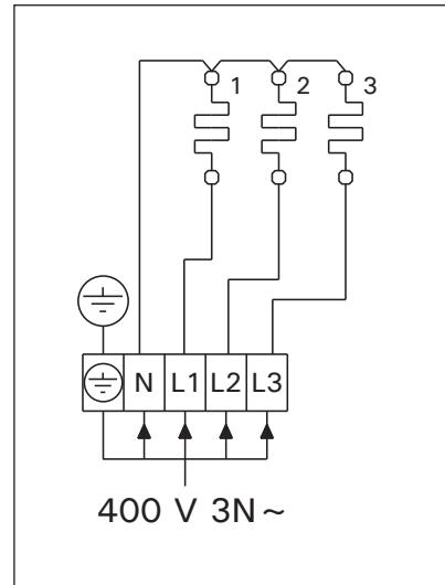
14. zīm. Elektrības pievienošana ME krāsnij
