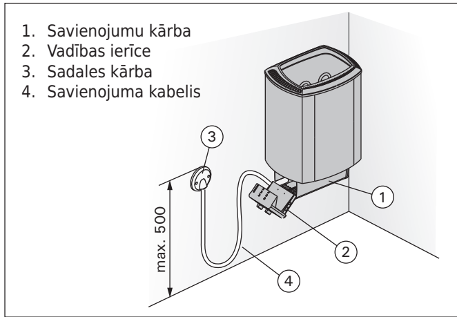
10. zīm. Krāsns pievienošana un tās daļas
