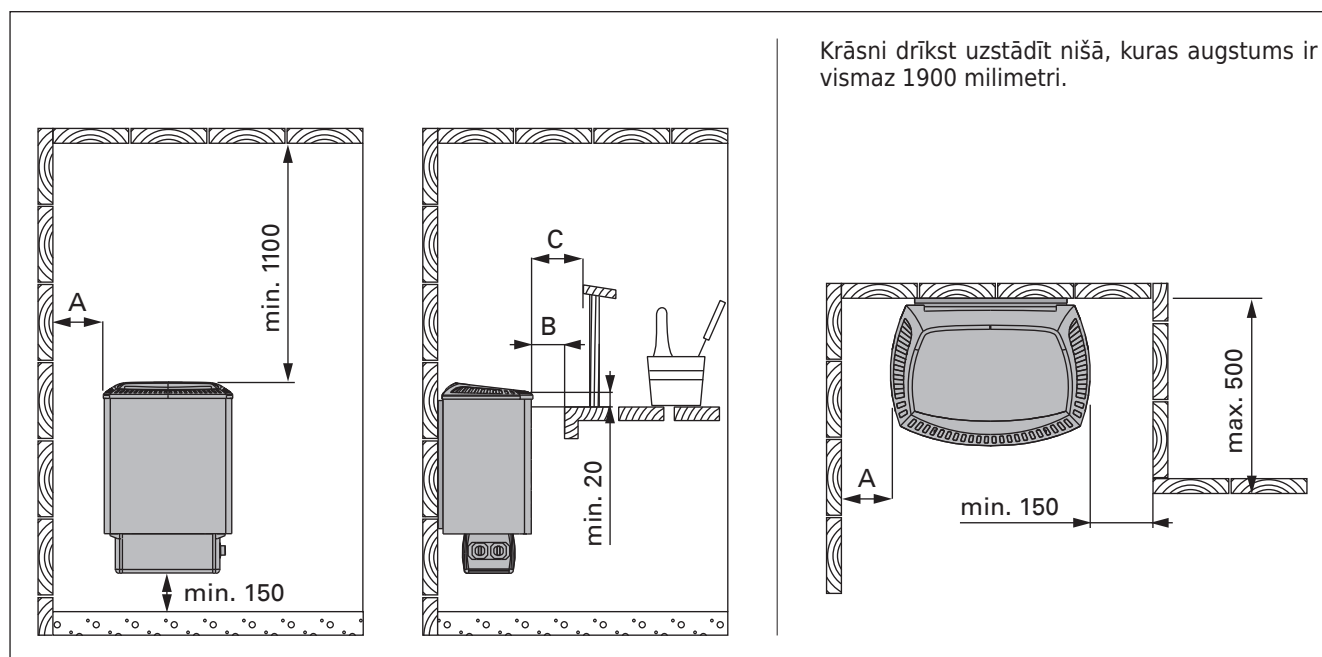
6. zīm. Drošības attālumi (visi gabarīti milimetros)
