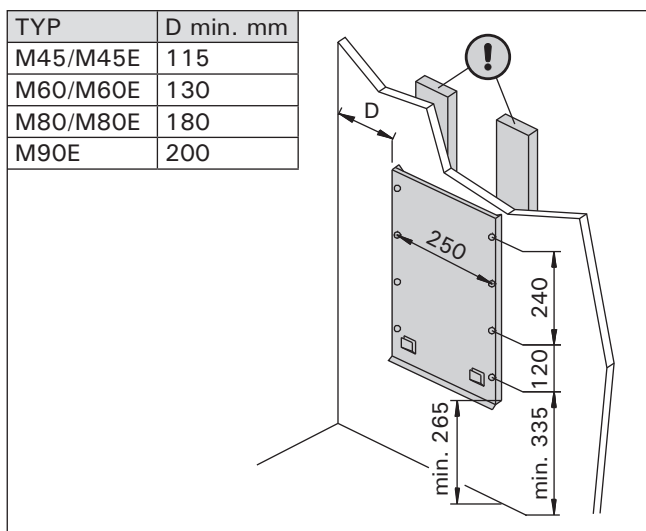
9. zīm. Krāsns piestiprināšana pie sienas (visi gabarīti milimetros)
