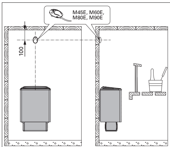
11. zīm. Sensoru uzstādīšana (visi gabarīti milimetros)
