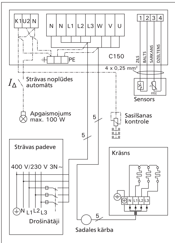
15. zīm. Vadības ierīces C150 un M-E krāsns elektriskie savienojumi
