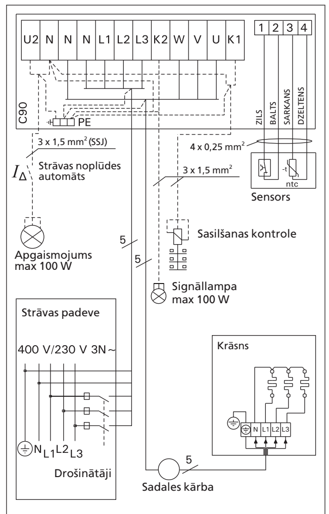
16. zīm. Vadības ierīces C90 un M-E krāsns elektriskie savienojumi
