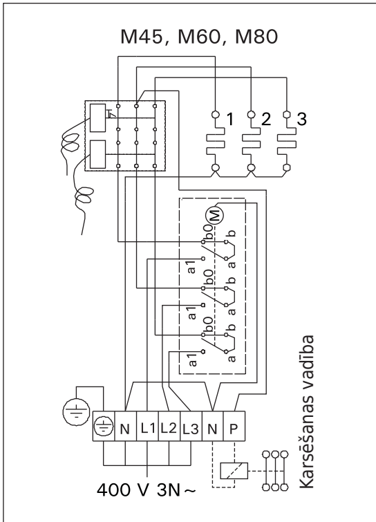
13. zīm. Elektrības pievienošana M krāsnij
